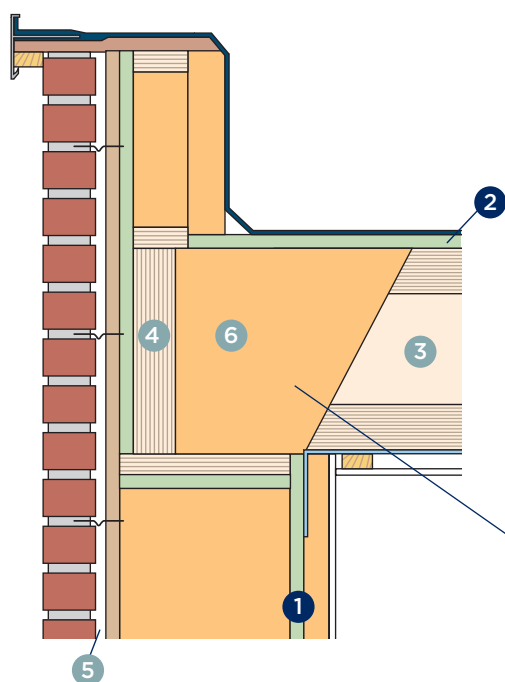
Jonction entre le mur et le toit plat
