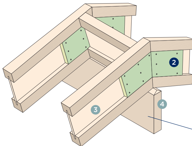
Poutre de faîte
