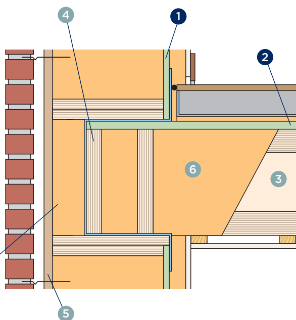
Sol avec jonction avec le mur Méthode de la plateforme
