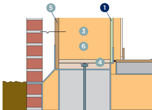
Jonction des fondations
