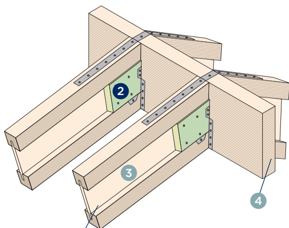
Jonction avec la poutre de faîte
